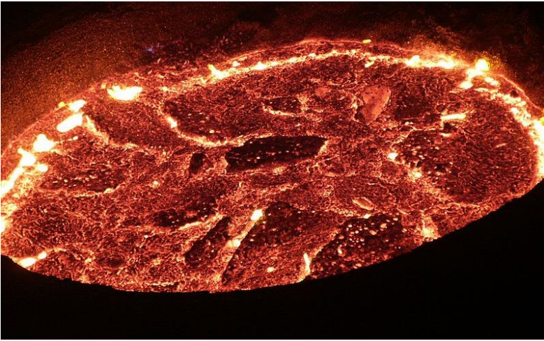
Resim 1. Eritilmiş ve cüruftan ayrılmış saf demir.
